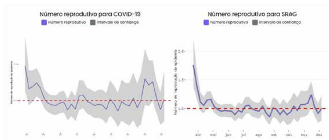
Gráfico 2 – Número Reprodutivo efetivo R_e para o Município de Osasco.
