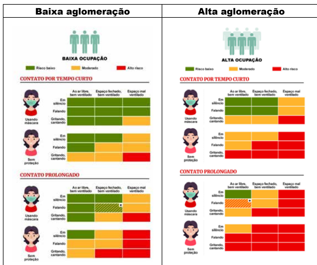
Figura 1 – Risco de transmissão de covid-19
