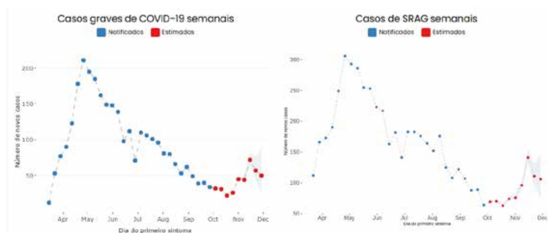
Gráfico 1 – Estimativa de casos graves de COVID-19 e SRAG em Osasco
